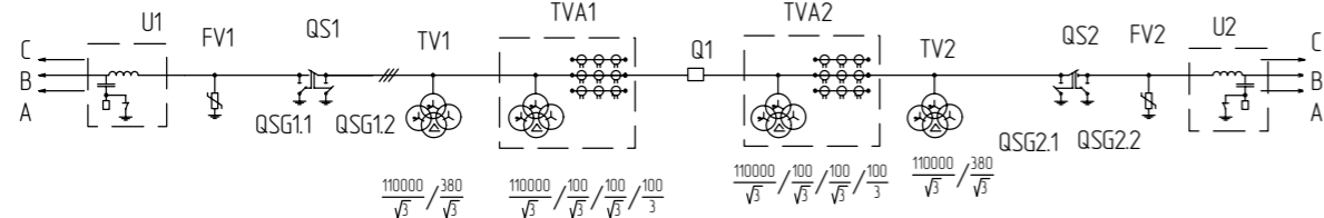
Схема электрическая главная МС-110
