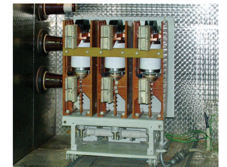
► Испытание выключателя ВРЗ в климатической камере
